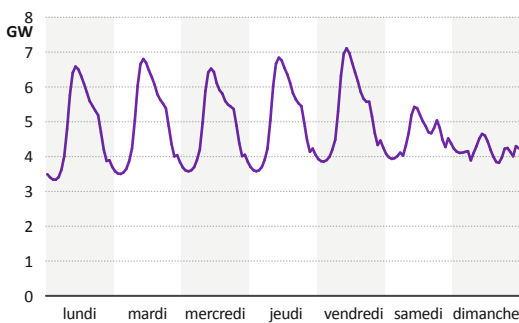
Consommation d'entreprises tertiaires raccordées en BT > 36 kVA pour une semaine froide en hiver
