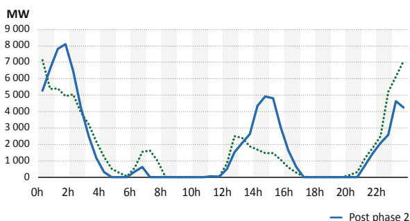
Hiver - effet des Heures Creuses - Simulation post phase 2***
