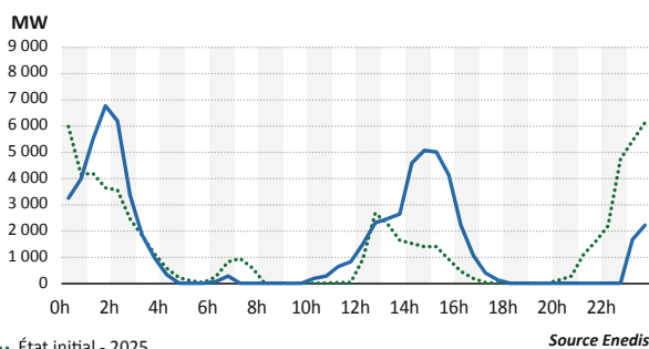
Été - effet des Heures Creuses - Simulation post phase 2
