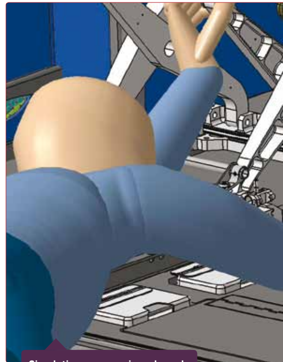
Simulation ergonomique lors de la conception du Falcon 7X en utilisant un logiciel Dassault Systèmes.
